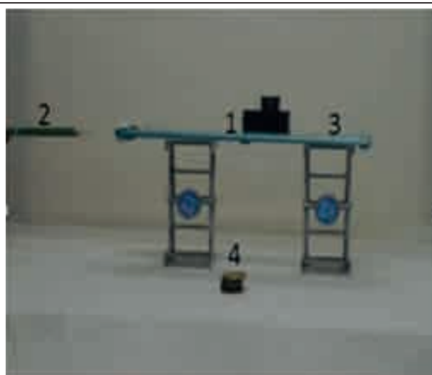
Figura 1. Rozamiento - parte 1. Áreas diferentes.
